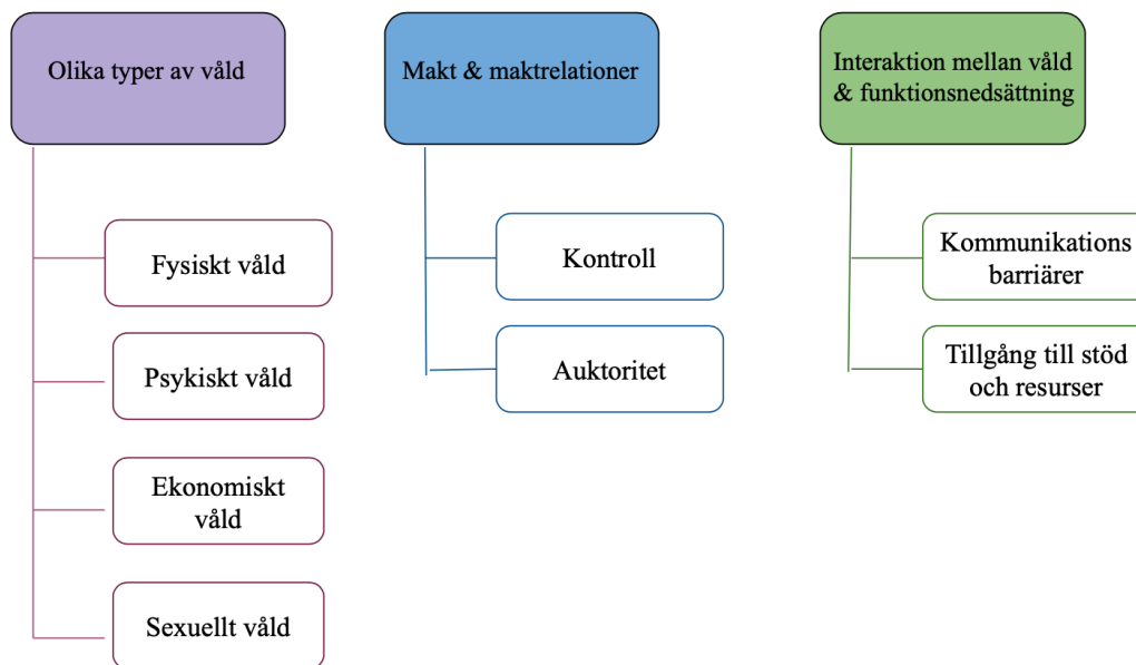
Figur 2: Tematiskt schema
